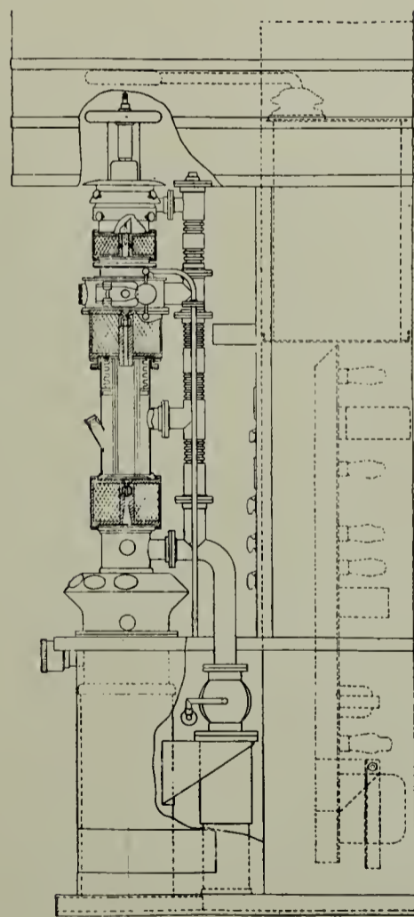
4—Esquema del microscopio electrónico. (Su altura es de unos 2,50 metros).
